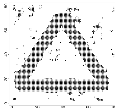
Figure 2. Edge Points
